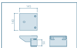
各ディスプレイアーム取付用 クルーズ Cタイプ専用クランプ金具 MY801X-Z637
